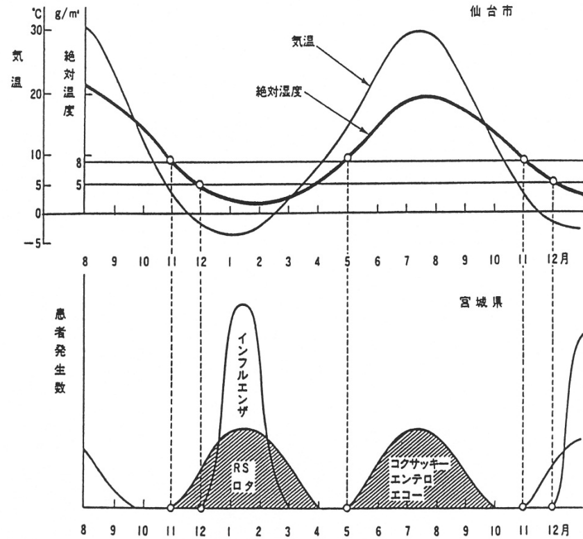
図2 かぜの流行と絶対湿度(空気中の水)
